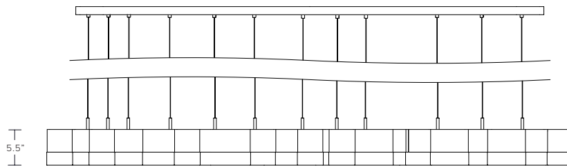
MULTI-MODULE CHANDELIER, 5 + 7 + 11 + 11
