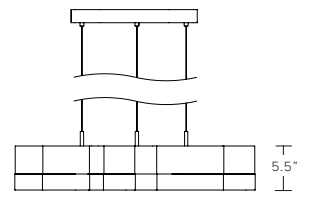
11 PC MODULE
